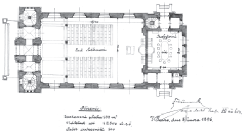
Náčrtek na stavbu evangelického reformovaného kostela v Mělníku
